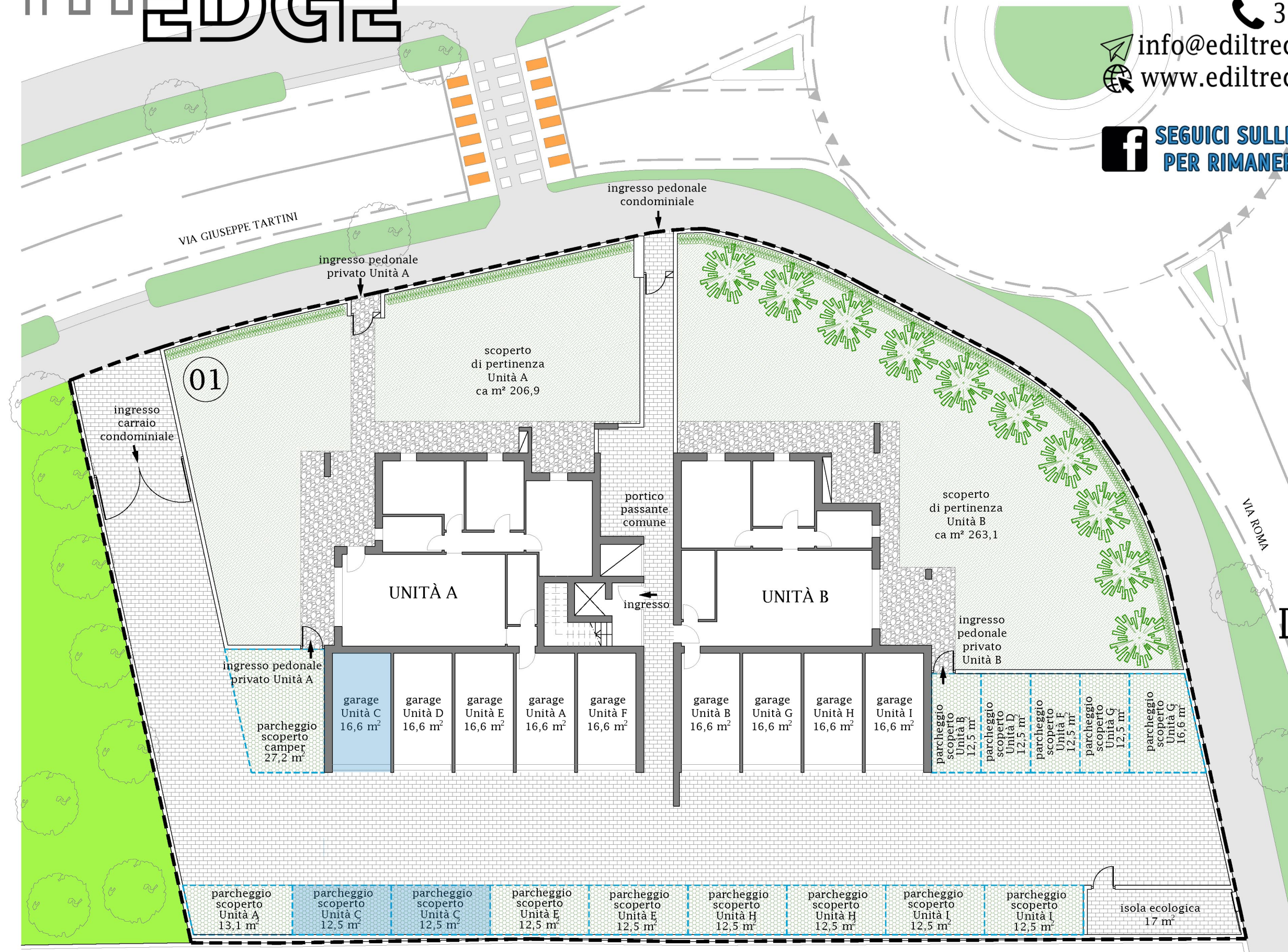
Planimetria sistemazione aree scoperte Scala 1:200
